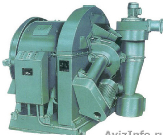
Барабанный дробемет
